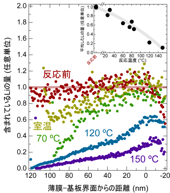
図2 各温度でのLiイオンの脱離反応前後の薄膜に含まれるLi量
