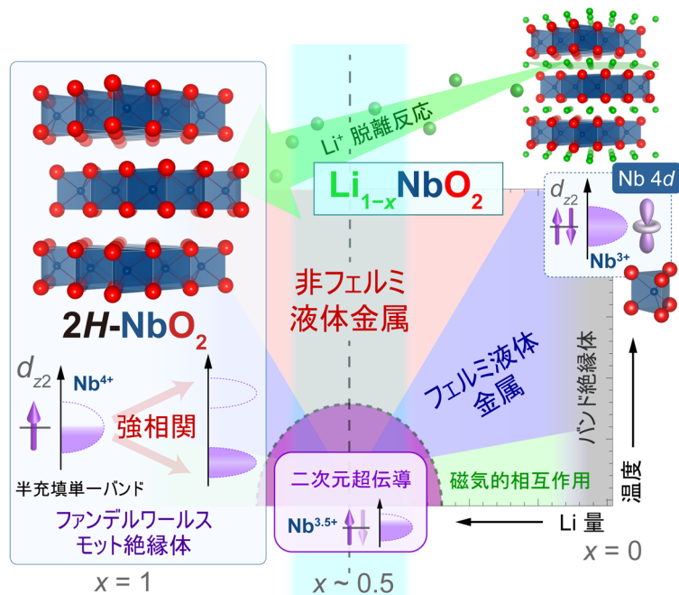
図3 Li イオンの脱離反応に伴う \text{Li}_{1-x}\text{NbO}_2 の電気的特性の変化
