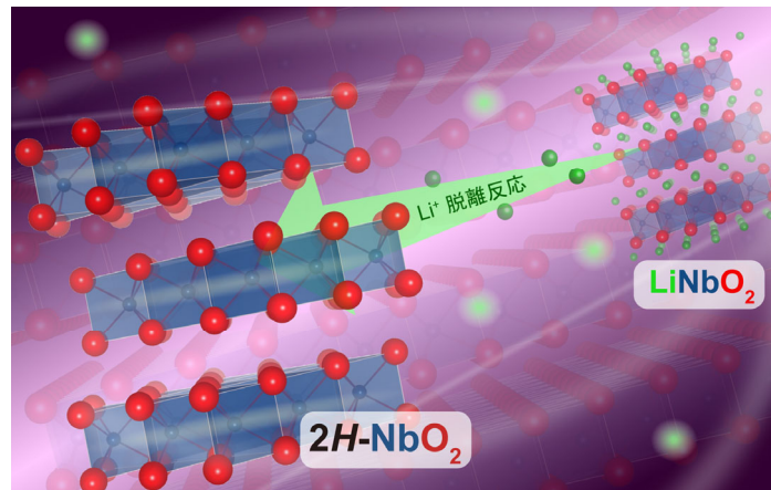
図1 \text{LiNbO}_2 から 2H\text{-NbO}_2 を合成する戦略
